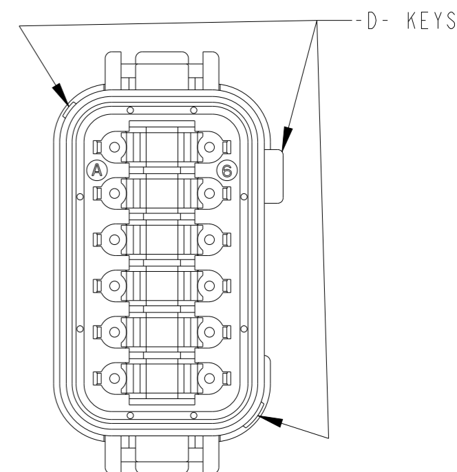
DT06-12SD-CE05 KEY ARR. -D- COLOR: BROWN
