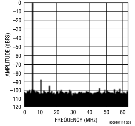
LTM9011-14: 8k Point FFT, f_{IN} = 5\text{MHz} , -1\text{dBFS} , 125\text{Mpsps}
