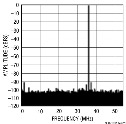
LTM9010-14: 8k Point FFT, f_{IN} = 70\text{MHz} , -1\text{dBFS} , 105\text{Mps}
