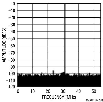
LTM9010-14: 8k Point FFT, f_{IN} = 30\text{MHz} , -1\text{dBFS} , 105\text{Mps}
