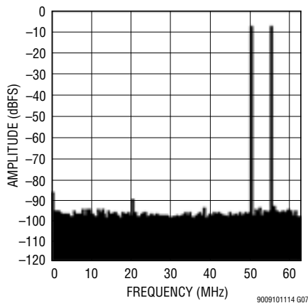
LTM9011-14: 8k Point 2-Tone FFT, f_{IN} = 70\text{MHz} , 75\text{MHz} , -7\text{dBFS} per Tone, 125\text{Mpsps}
