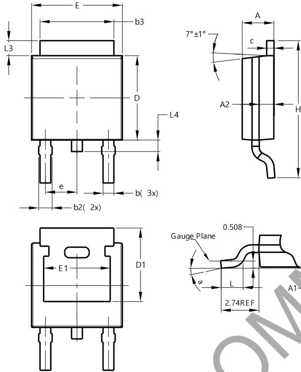
TO252 (DPAK)
